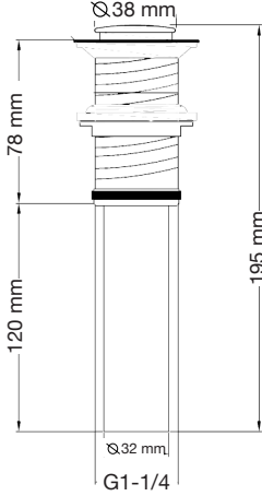
Cierre interior sin rebosadero Mod. 90.0154SR
