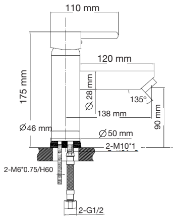
Monomando Alto Mod. 3210
