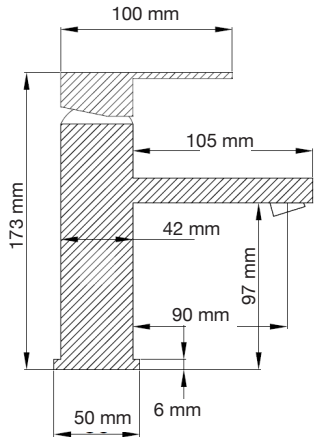
Monomando Bajo Mod. 28.0001
