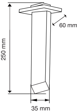
Brazo a Techo Negro Mod. 8403N
