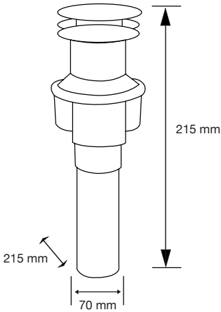
Cierre interior sin rebosadero Mod. 90.0154SR
