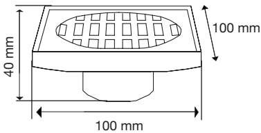
Coladera Rejilla latón Cromado Mod. 90.5001
