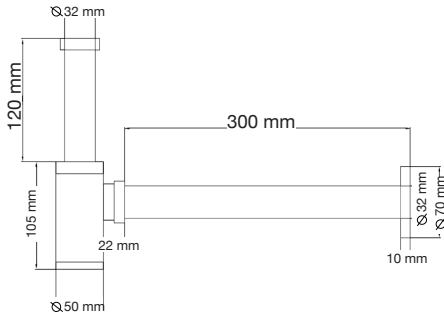
Sifón Recto Mod. 90.0093
