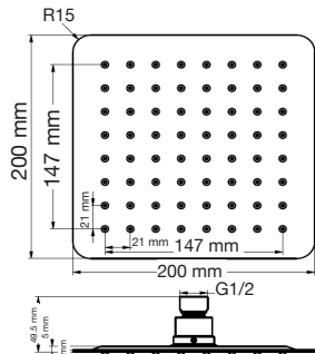
Regadera Odessa cuadrada Mod. 8640N
