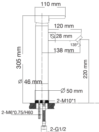
Monomando Bajo Mod. 3212
