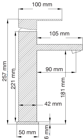
Monomando Alto Mod. 28.0002
