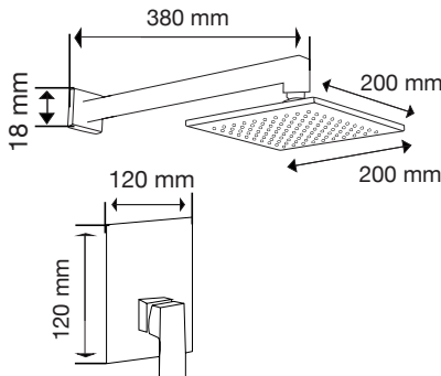
Kit Morán cuadrado Mod. 68.003
