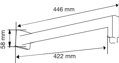
Brazo a pared regadera Odessa Mod. 8402N
