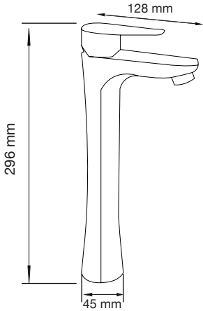
Monomando Alto Mod. 60.0002
