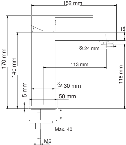
Monomando Bajo Mod. 75.1229
