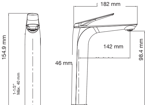
Monomando Bajo Mod. 78.0101G
