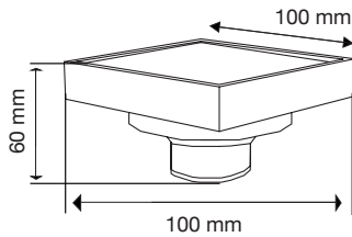
Coladera CLEAN cuadrada gold Mod. 90.5006G
