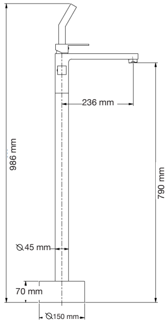
Monomando Bañera Lexus Mod. 8536
