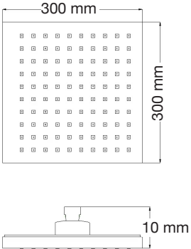
Regadera exterior Lexus Mod. 75.2340
