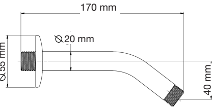
Brazo y Chapetón Mod. 5300000C
