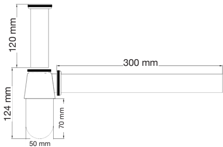
Sifón Botella Mod. 90.0007
