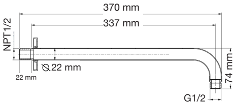
Brazo a Pared Mod. 5412200C
