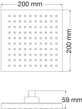
Regadera de teléfono Lexus Mod. 53.3011
