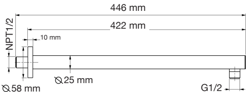
Brazo a Pared regadera de alta presión Mod. 5450401C
