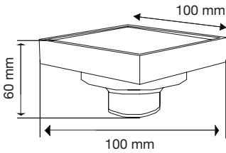
Coladera CLEAN cuadrada inox Mod. 90.5006I
