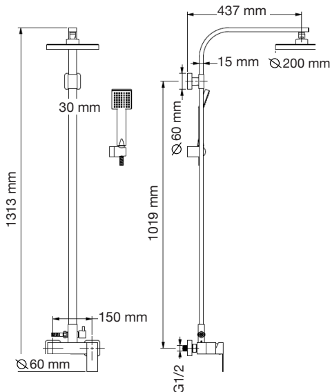
Kit Morán cuadrado Mod. 68.003
