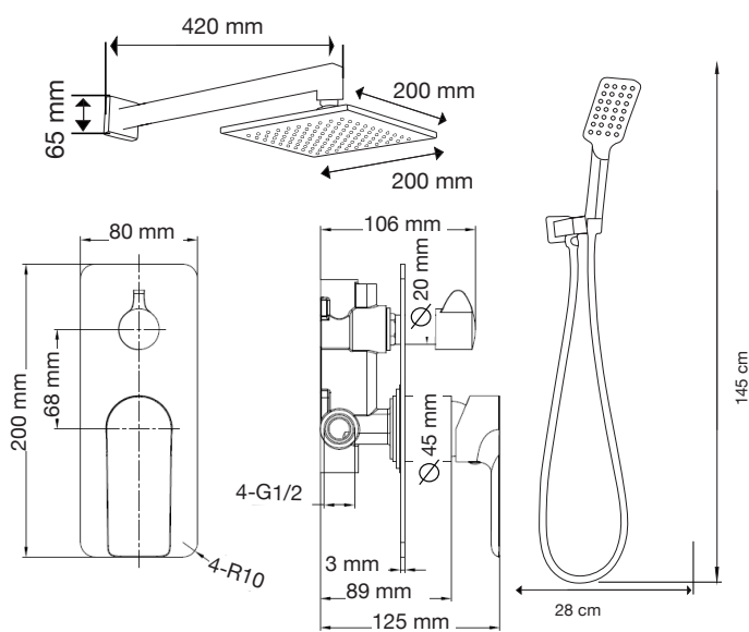
Kit Bonati cuadrada Mod. 78.0103G
