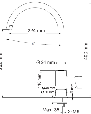
Monomando Fregadero New York Mod. 83.0201
