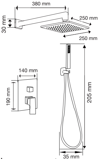
Kit Morán cuadrado con teléfono Mod. 68.002C
