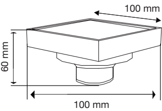
Coladera Cuadrada Latón Satinado Doble vista Mod. 90.5023A
