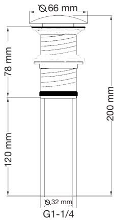
Cierre exterior sin rebosadero Mod. 90.0155SR
