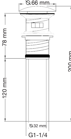
Cierre exterior con rebosadero Mod. 90.0055CR
