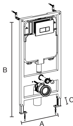
BOTÓN A MURO A: 530 mm B: 1112 mm C: 80 mm
