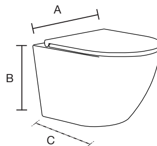
SANITARIO A: 365 mm B: 355 mm C: 480 mm
